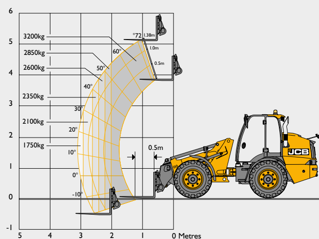
TM320 / TM320S
